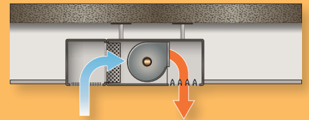
Zwischendeckenmontage
