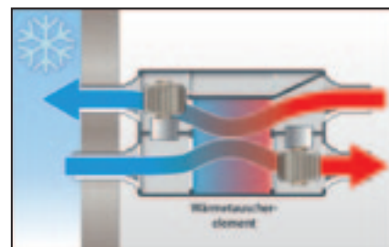
Winterbetrieb
