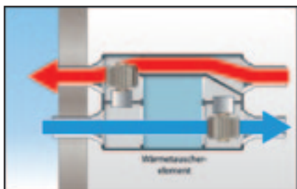
Bypass-Betrieb
