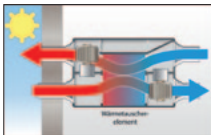
Sommerbetrieb
