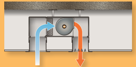
Zwischendeckenmontage
